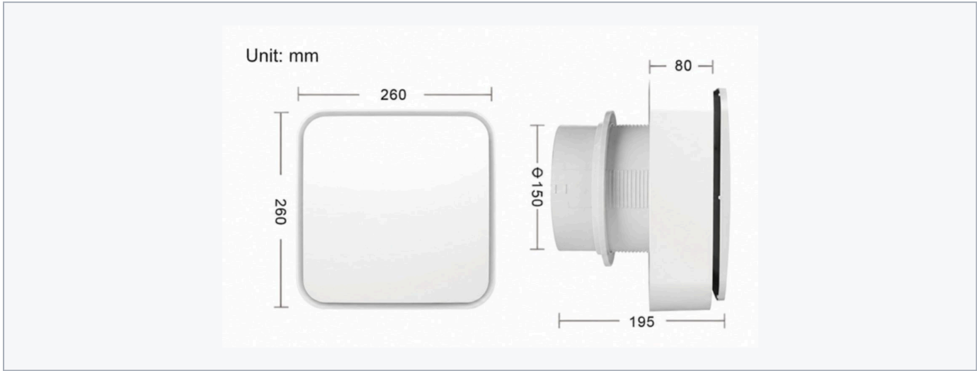
Fig. 2 A = largura · B = altura · C = profundidade do corpo · D = profundidade total com a conexão
