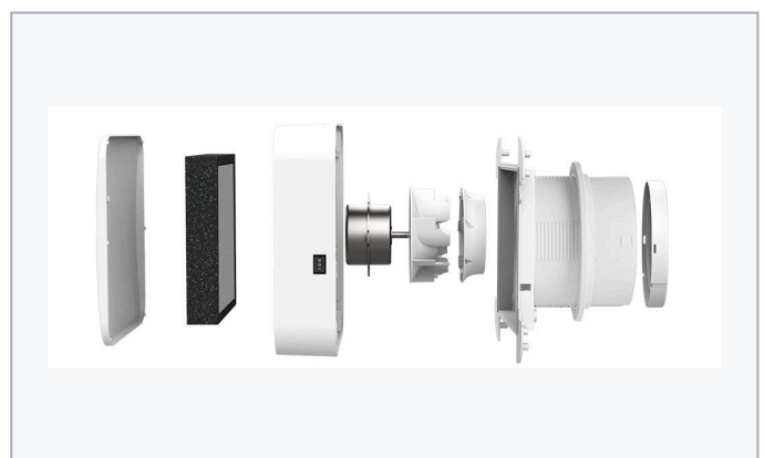
Fig. 1 Painel · filtro HEPA · liga/desliga · motor · rotor · conexão para duto
